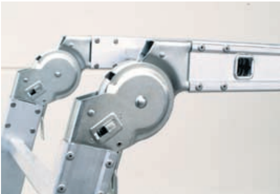
Bild 50: Sperrstellung der Gelenke
