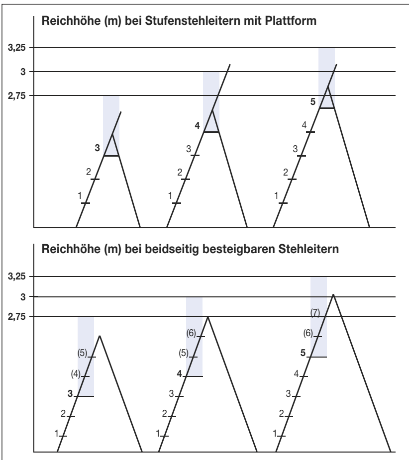
Bild 39: Reichhöhen
